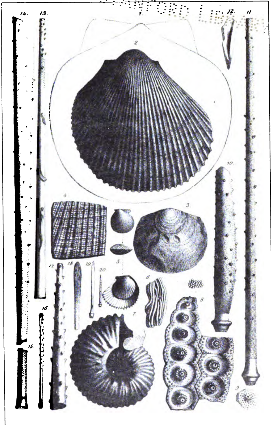
Owenstedt, Jura.
